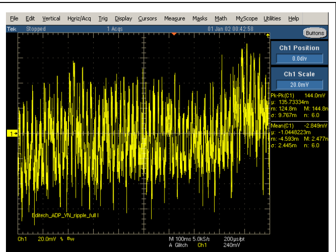
Fig. 4: PP_PWR_IN
